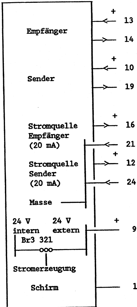
25polige Buchse Stift-Nr.
