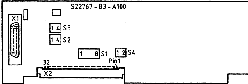
Bild 14 Lage der Betriebsartenschalter S1, S2, S3 und S4 auf der SAP-S3
